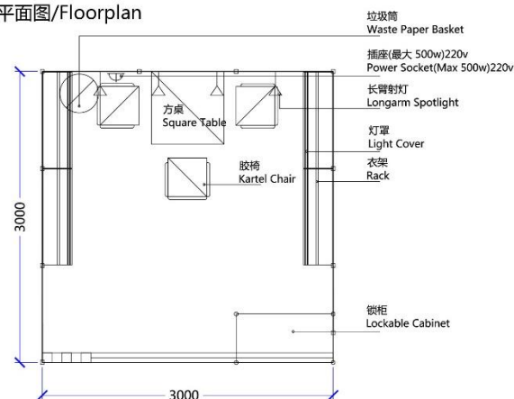
平面图/Floorplan
