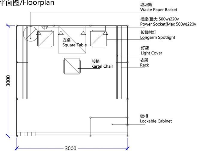
平面图/Floorplan
